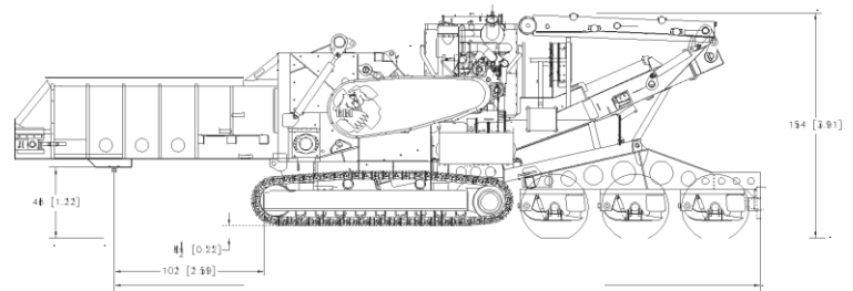
Транспортное положение
